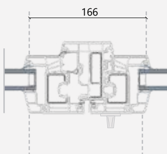
sezione B-B1
