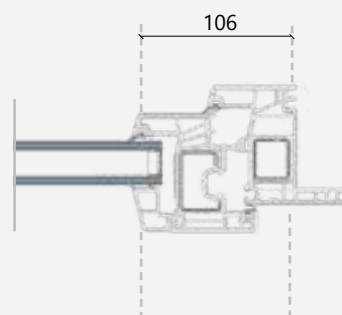
sezione C-C1
